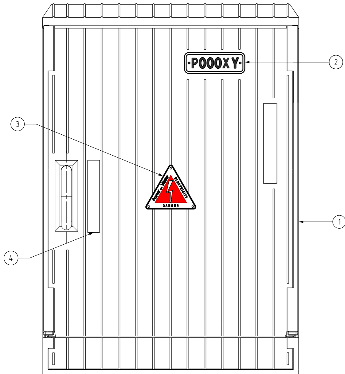
PILLAR SIGN LAYOUT SCALE N.T.S.
