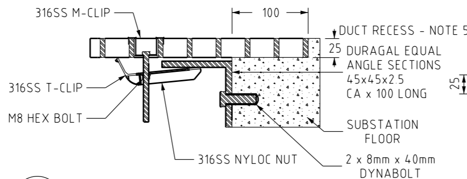
LOCKED POSITION SECTION B N.T.S.
